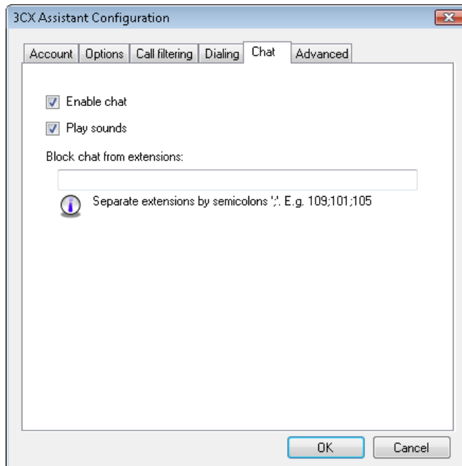
Рис. 3. Настройка чата
