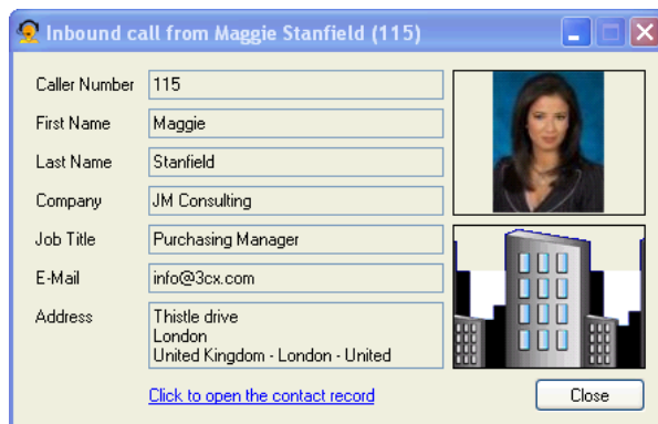
Рис. 33. Всплывающее окно
