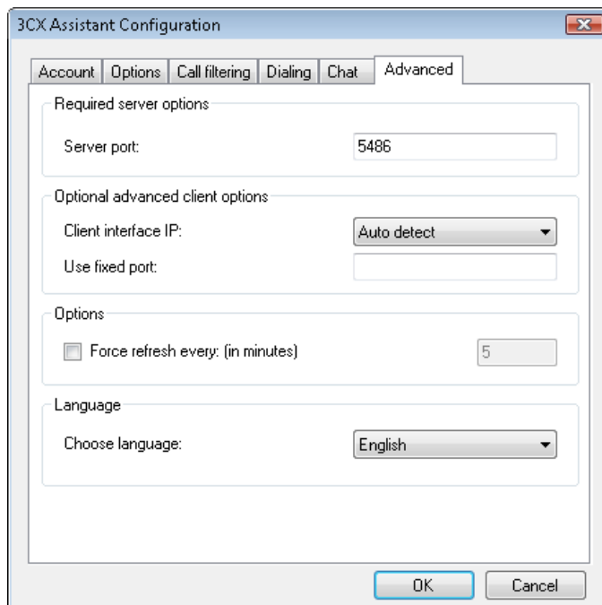
Рис. 4. Дополнительные настройки
