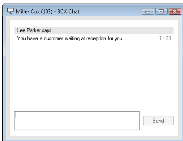
Рис. 2. Текстовый чат
