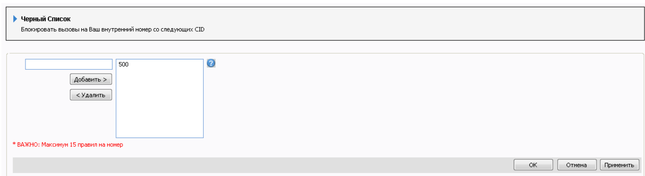
Рис.27. Черный список
