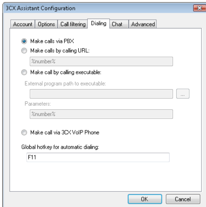
Рис. 2. Настройки вызовов
